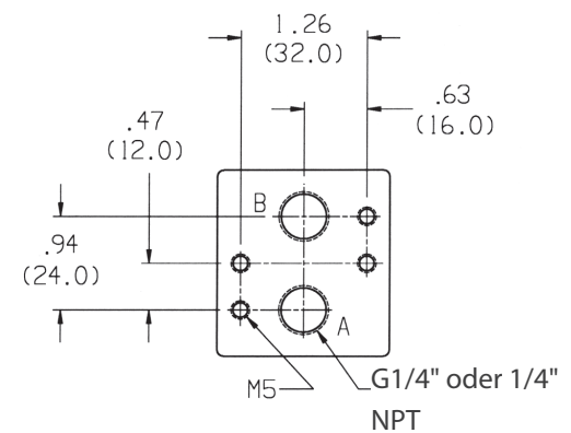
Magnetventilschnittstelle
