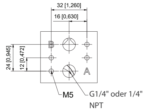
Magnetventilschnittstelle
