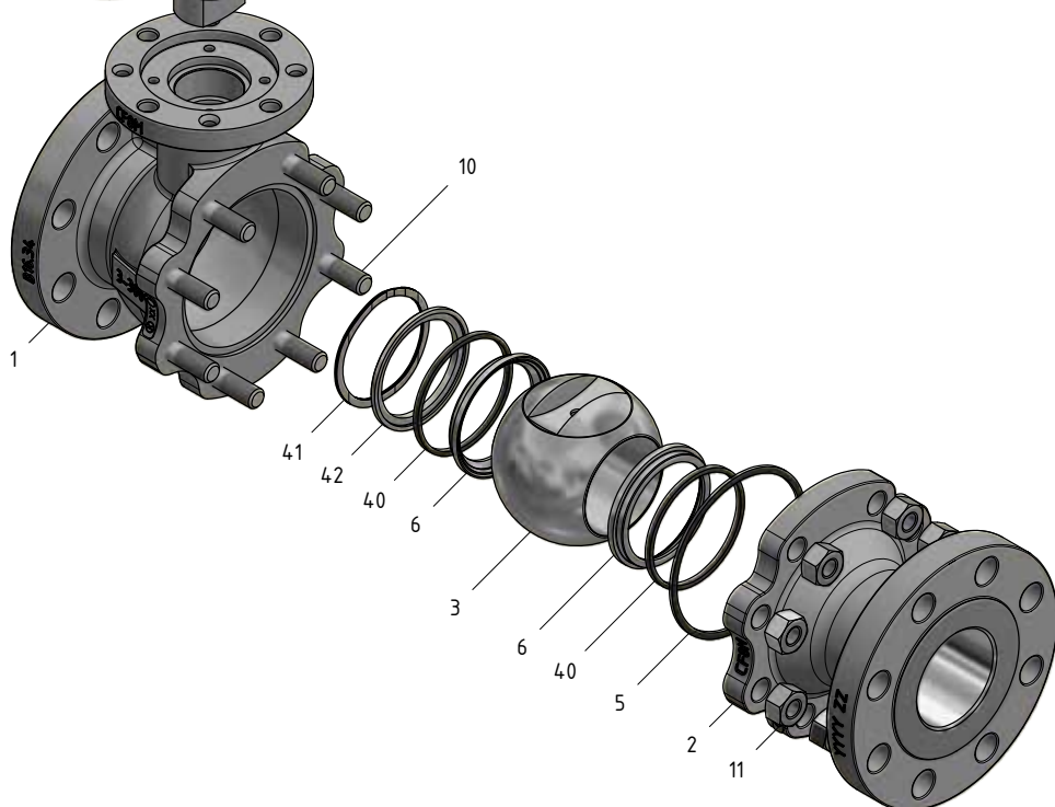
6" 300 级浮球设计, 含关键连接项目 16
