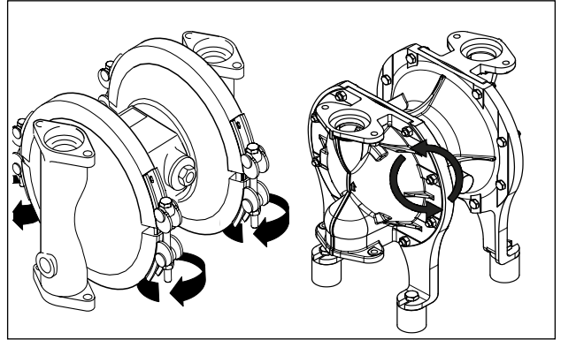
Res. 9: Germe bantlarını açıp civataları sökün (vidalı pompa modelinde).
