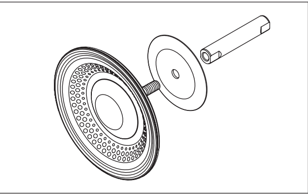
Res. 14: Montaj noppedE4® diyaframları.
