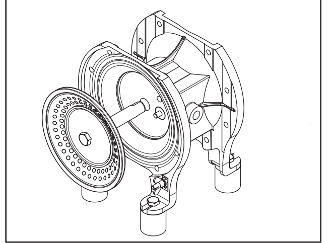
Res. 21: Diyaframı piston kolu yardımıyla çıkartmak
