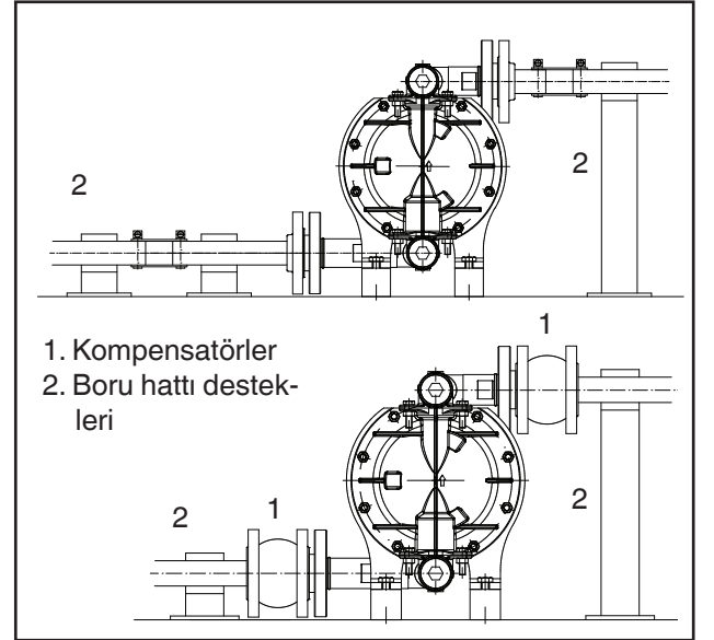
Res.3: Diyafram Pompaların Kurulumu
