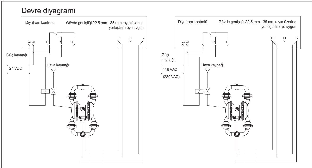
Res. 6: Sızıntı sensörleri için devre diyagramı
