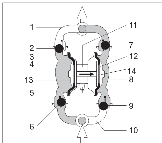
Рис. 2: Конструкция насоса
