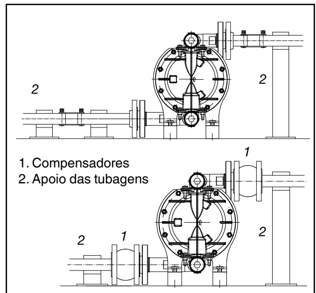
Fig. 3: Proposta de montagem para a bomba de diafragma
