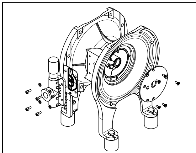
Abb. 23: Bomba DH com válvula de comando AirSave
