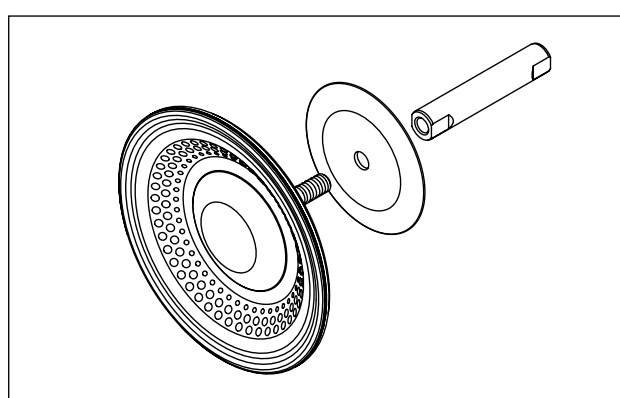
Fig. 14: Montagem da membrana nopped E4®.
