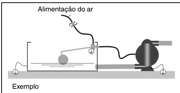
Fig. 26: Aviso de instalação do comando de nível
