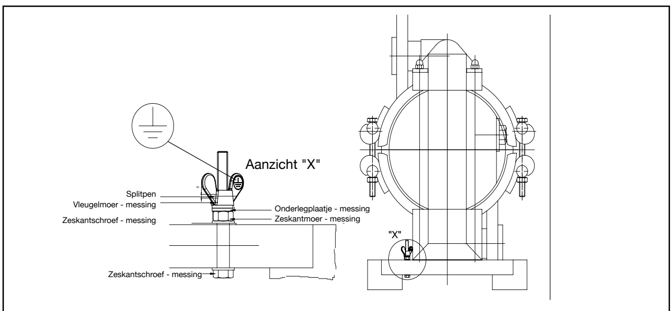
Afb. 5: Aardingsschroef
