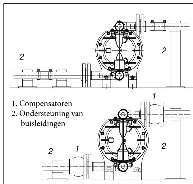
Afb. 3: Opstellingsvoorstel voor membraanpomp
