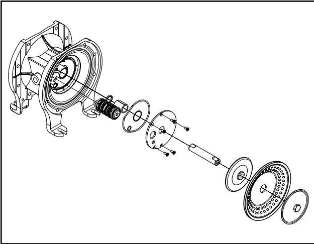
Afb. 22: DH-pomp met inwendige regelklep
