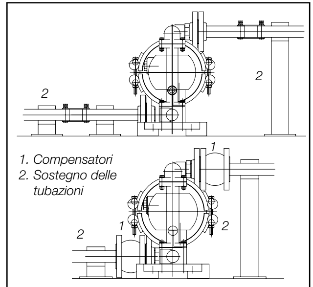
Fig. 3: Proposta di disposizione della pompa a diaframma
