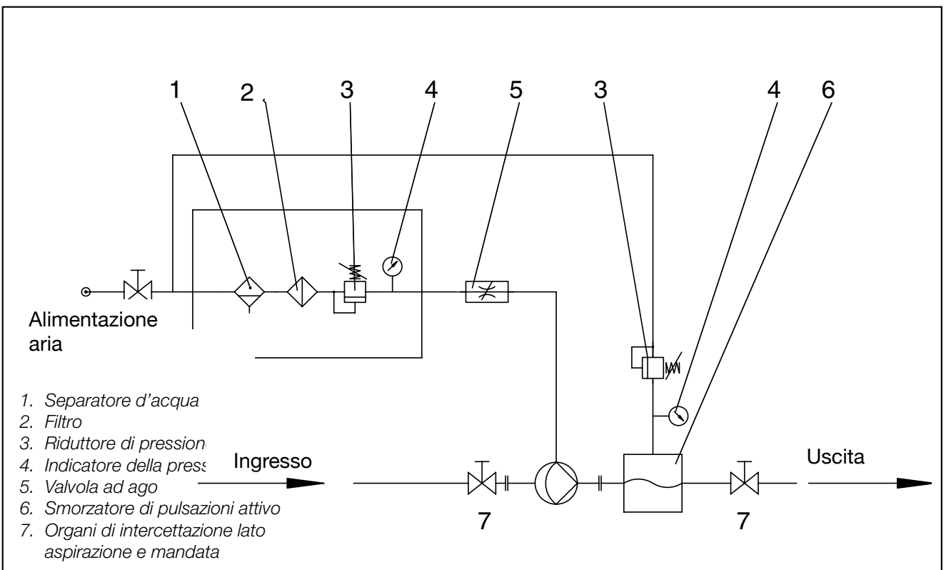
Fig. 4: Esempio di installazione della pompa
