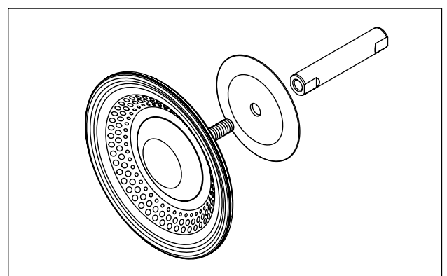
Fig. 14: Montaggio del diaframma noppedE4®.
