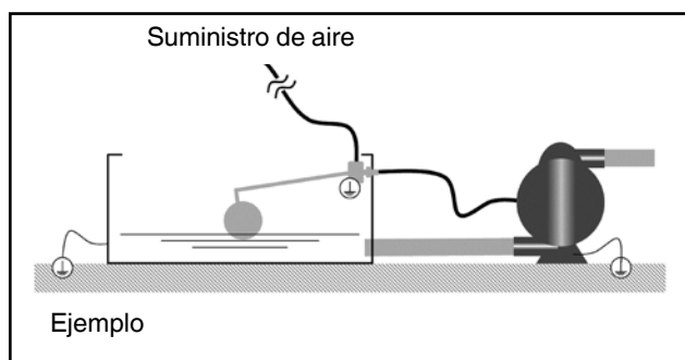
Fig. 24: Indicaciones de instalación del control de nivel
